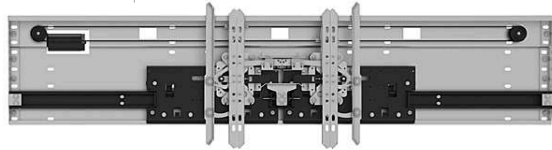
2 Panelli Merkezi Kapı Mekanizması 2 Panel Central Landing Door Mechanism
